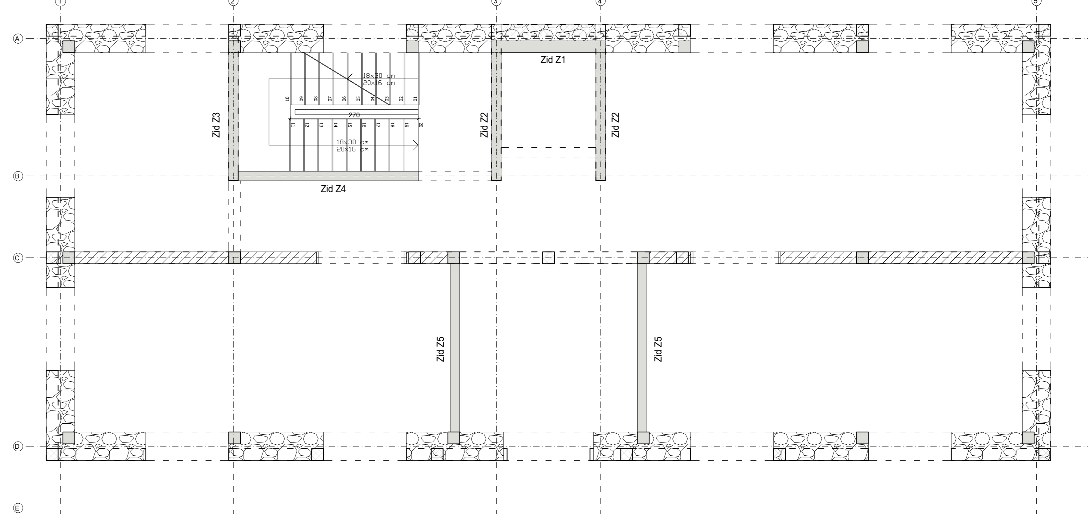
Pregledni plan zidova prizemlja mj 1:50, C25/30, cnom=2,5 cm
