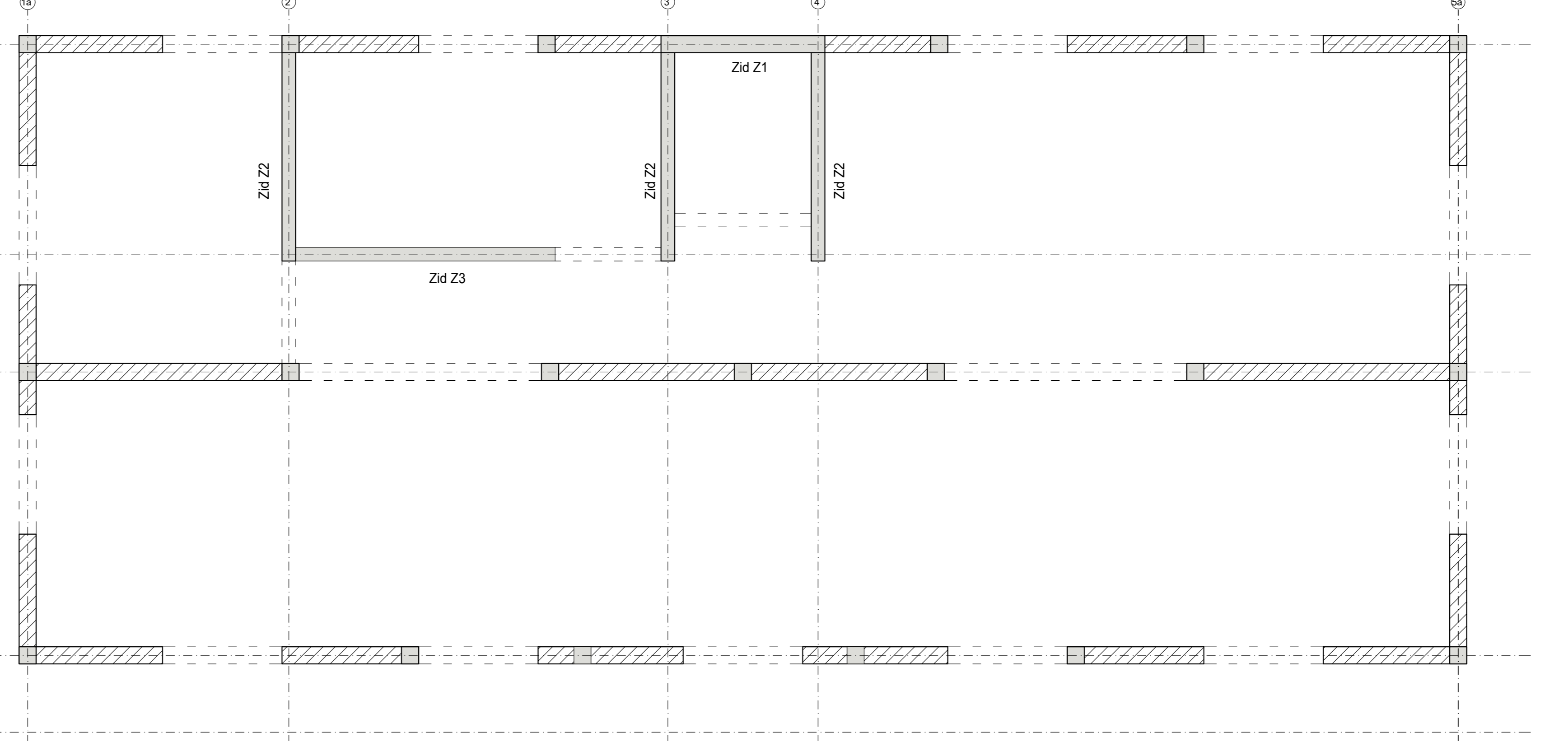
Pregledni plan zidova 1. kata mj 1:50, C25/30, cnom=2,5 cm
