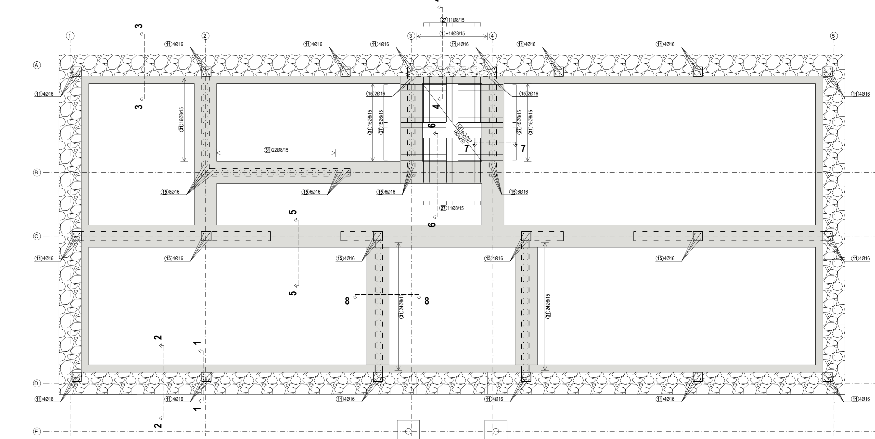
Armatura temeljnih traka - Podna ploča lifta i ankeri mj 1:50, C25/30, cnom=4,0 cm
